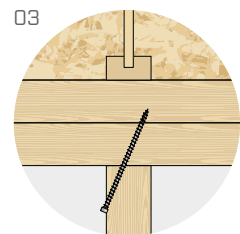
Unión montante-vigueta transversal con un único conector inclinado
